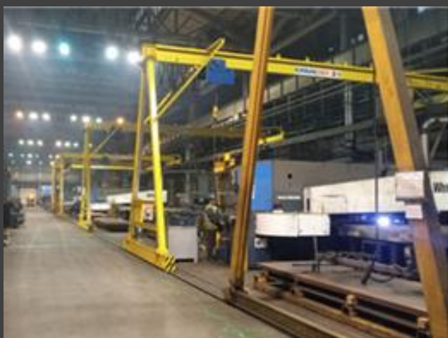
Ручные мобильные козловые краны
